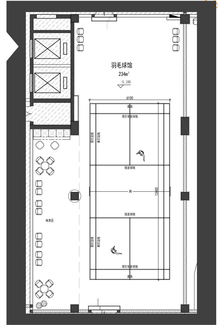
羽毛球馆设计
